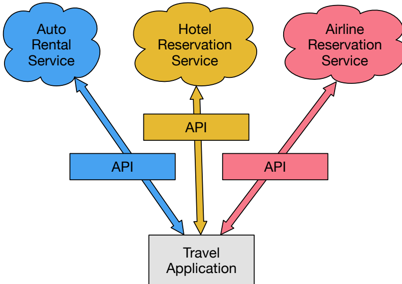
Abbildung 13.2: Serviceorientierte Architektur
