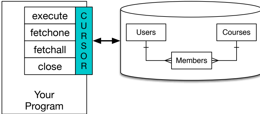
Abbildung 15.2: Ein Datenbankcursor
