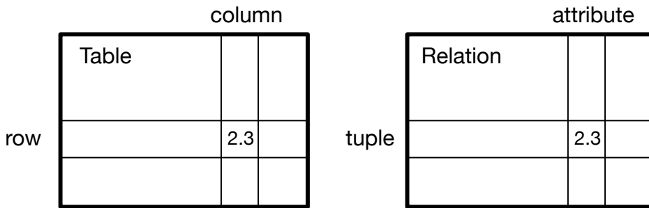
Abbildung 15.1: Relationale Datenbanken
